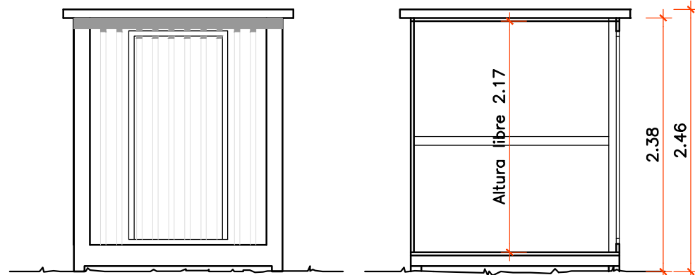
ALZADO FRONTAL
