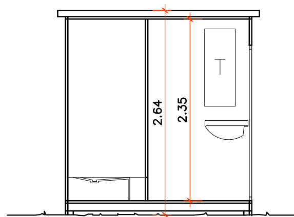
SECCIÓN A-A'
