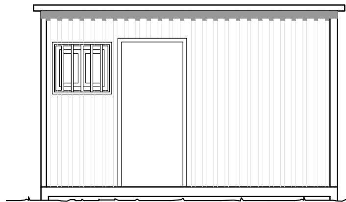
ALZADO FRONTAL
