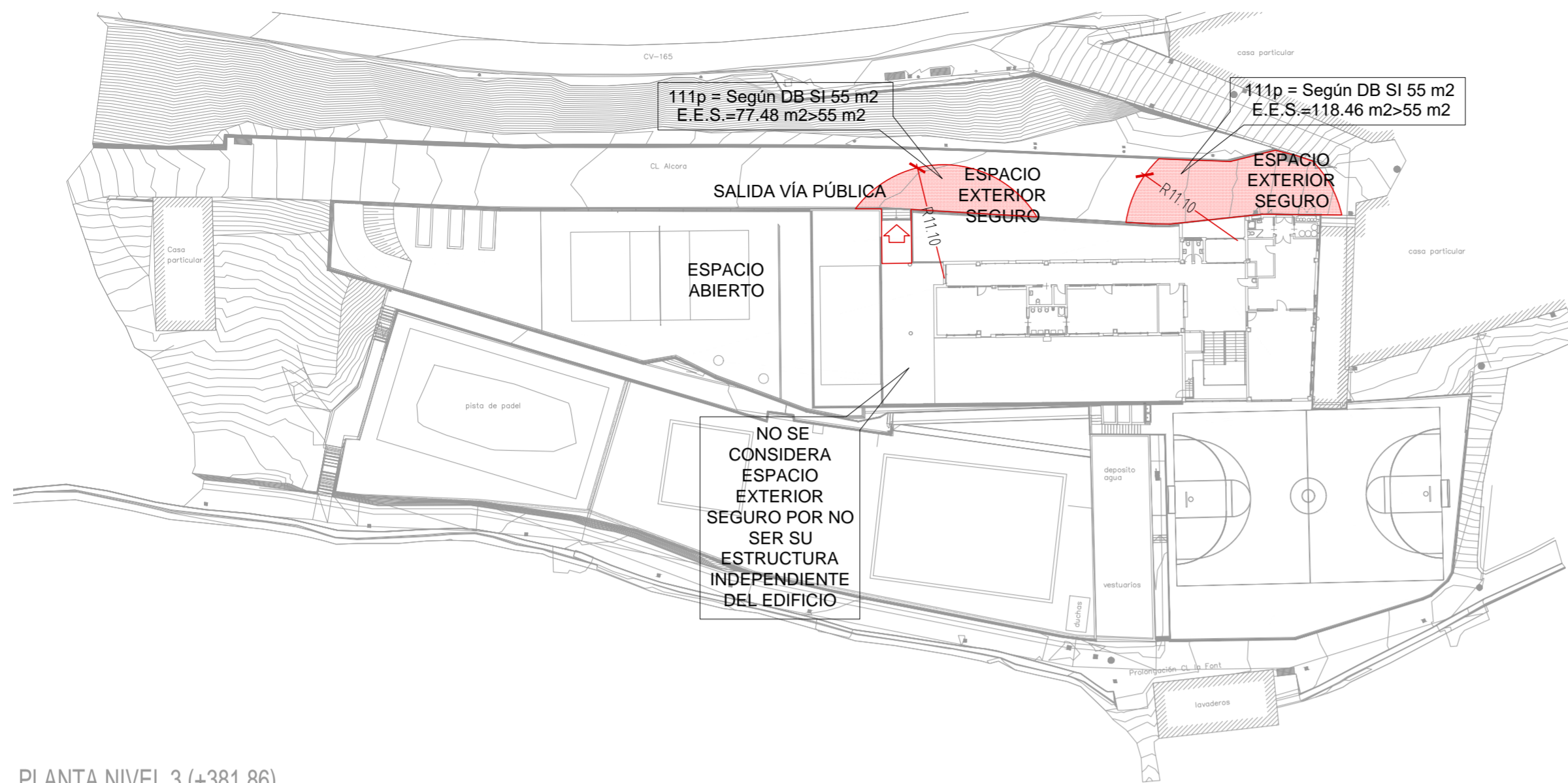
PLANTA NIVEL 3 (+381.86)
