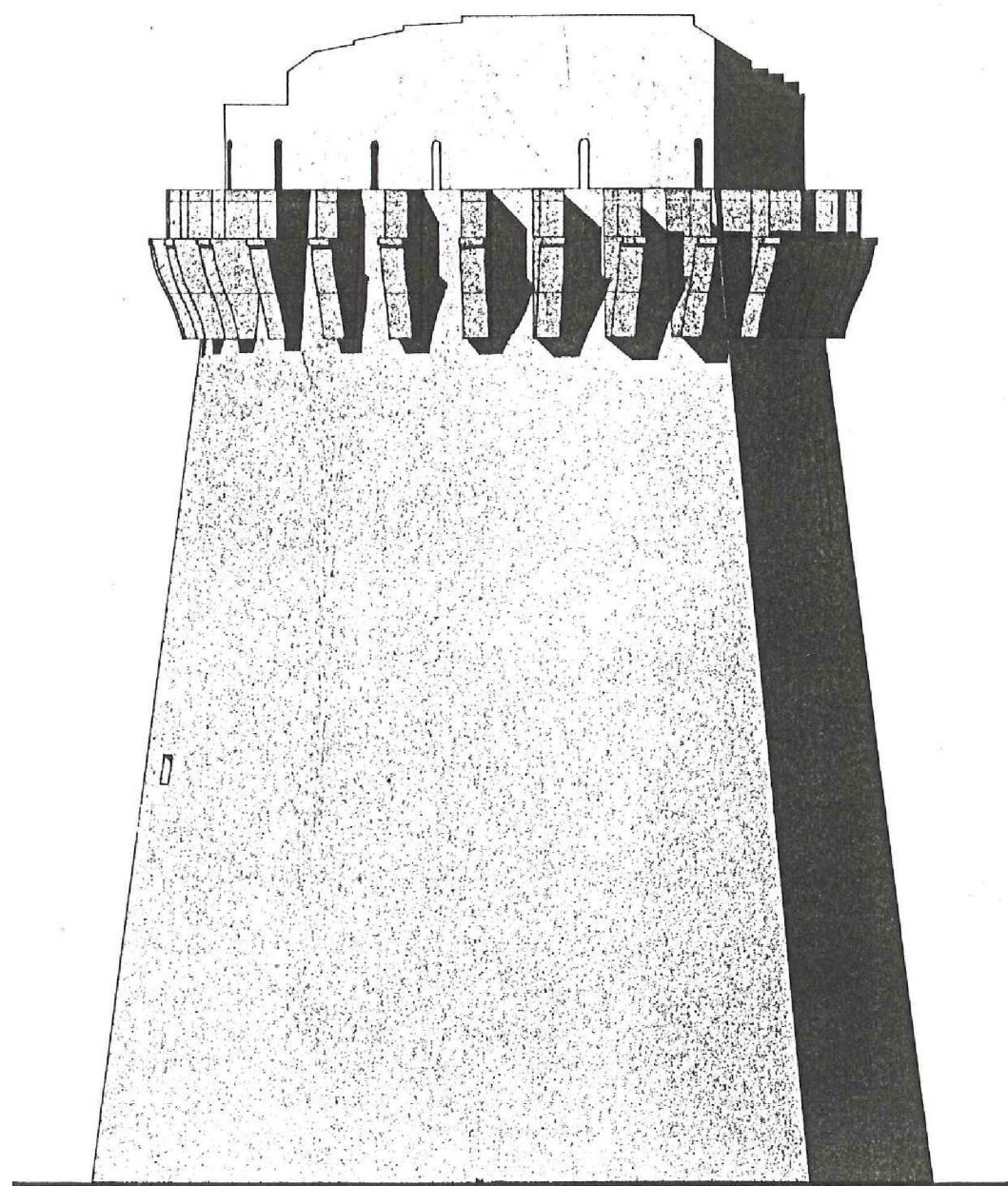
alzadoSUR
