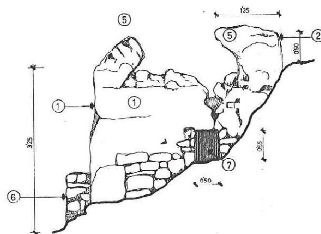
ALZADO LATERAL A
