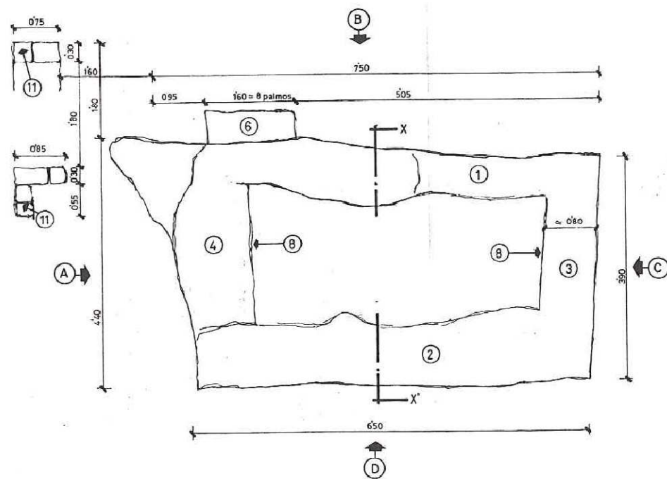
PLANTA DEL ALJIBE
