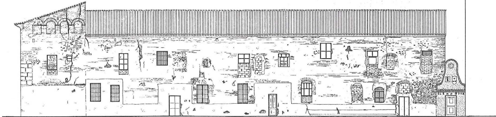
ALZADO CALLE JOSE ITURBI
