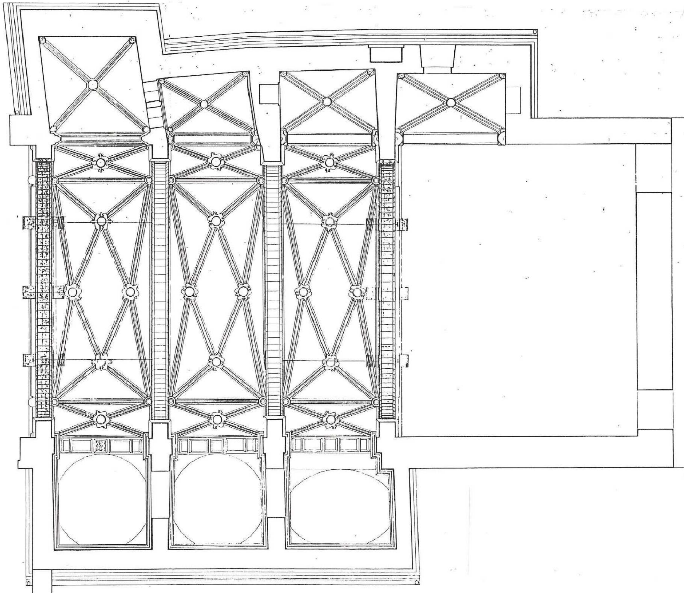
PLANTA ZENITAL
