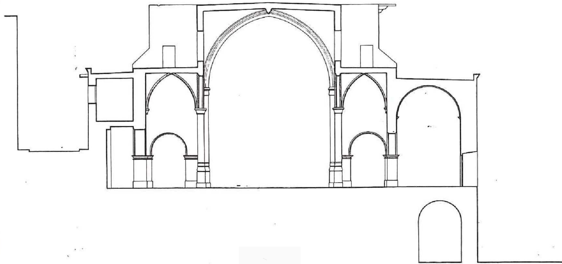
SECCIÓ TRANSVERSAL A
