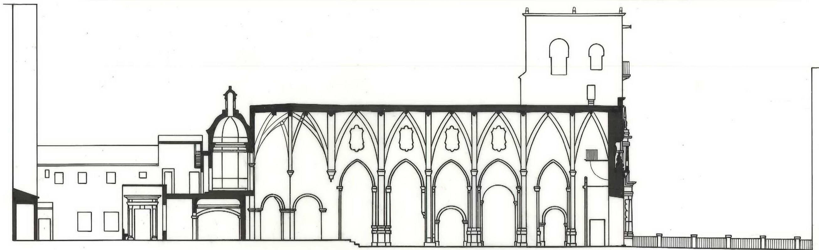
SECCIÓ LONGITUDINAL
